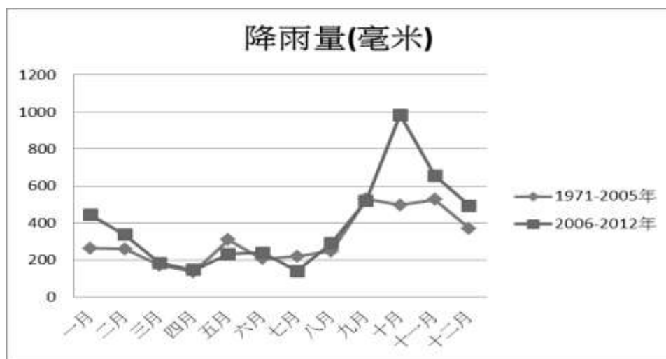
圖 3：蘇澳測站長短期降水量比較
