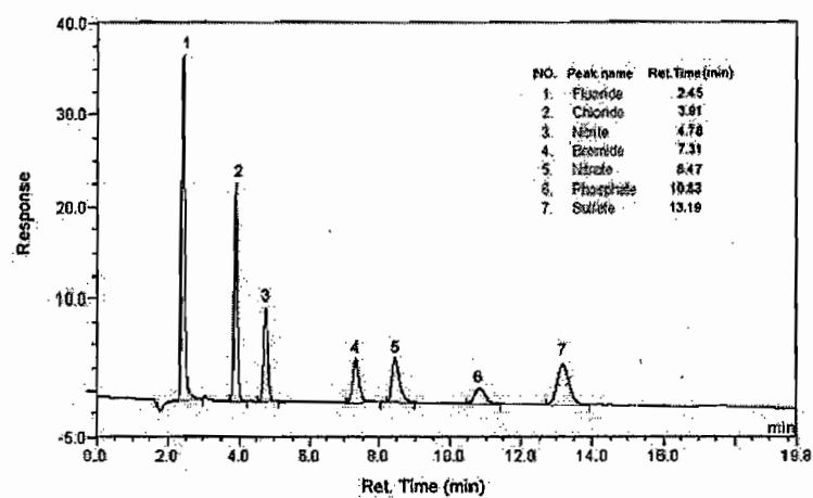
圖 七種陰離子標準品層析圖譜 (移動相溶液: 0.0003\text{ M NaHCO}_3 - 0.0027\text{ M Na}_2\text{CO}_3 , 流量: 1.5\text{ mL/min} 等速沖提, 層析管 Dionex AG12A plus AS12A, 各離子之濃度 5\text{ mg/L} , 注入體積 20\text{ }\mu\text{L} )
