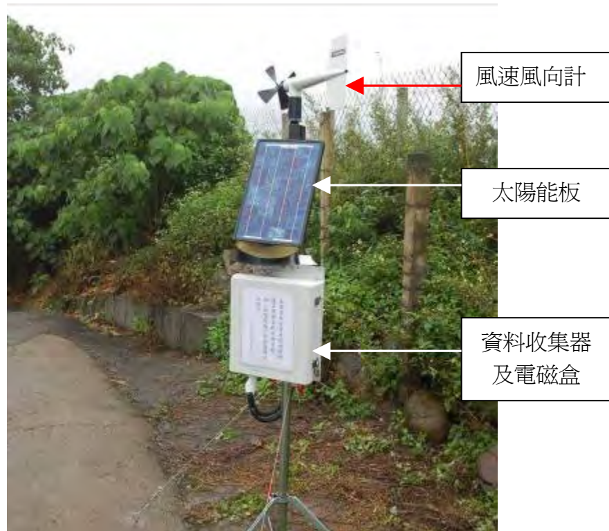
圖 19 九九峰自然保留區東側氣象測站照片（座標 230889,2657921）
