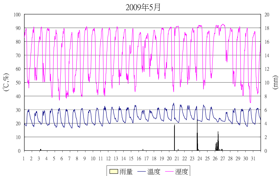
圖 39 2009 年 5 月東側氣象資料統計圖
