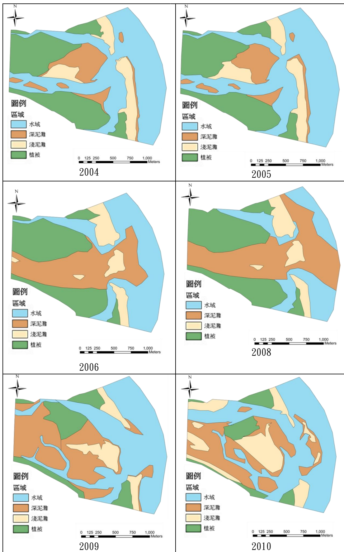
圖 8：蘭陽溪口 1996-2015 年間地形判識圖（續）
