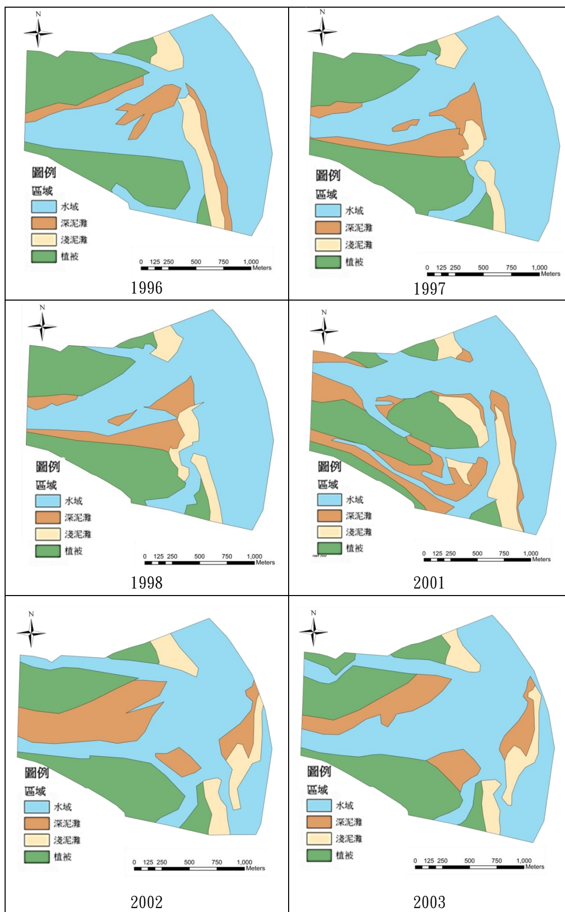
圖 7：蘭陽溪口 1996-2015 年間地形判識圖
