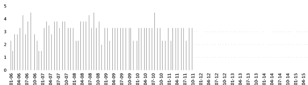
河川汙染指標(RPI) (2006/01-2015/07)
