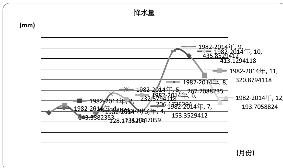
圖 3：宜蘭測站長期期降水量 (資料來源：中央氣象署，本計畫繪製)
