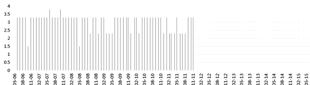
河川汙染指數(RPI) (2006/01-2015/07)
