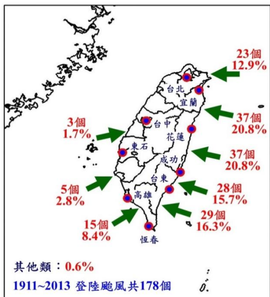
圖 4：颱風登陸地點之分段統計(1911~2013 年) 4
